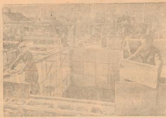
Ленинград. В районе проспекта Энгельса началось строительство первых в городе адлиторборных домов. Стены здания собираются на месте стройки из готовых бетонных панелей. Пространство между панелями заливается бетоном. Внутренние перегородки, балки, фризмы и карнизы также монтируются из заранее отлитых бетонных деталей. При отливке бетонные фасадные плиты сразу же отслаиваются. Это ликвидирует фасадные работы на стройке.
