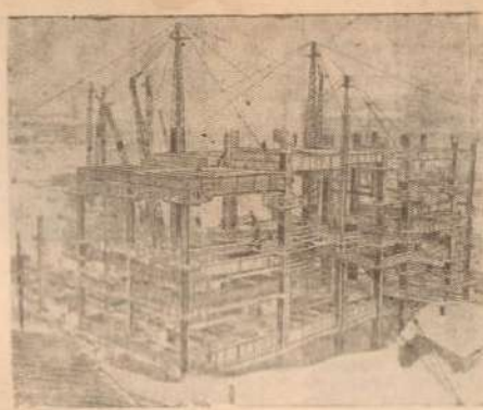
Первые стальные конструкции металлического каркаса нижней части здания Дворца Советов. Фото Г. Шарокова. Фото-кинем ТАСС.
