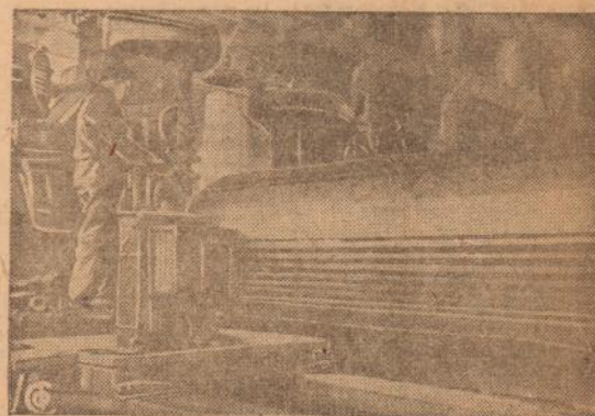
НА СНИМКЕ: Фрезеровка ротора турбогенератора на гигантском фрезерном станке. Вес ротора около 55 тонн.
